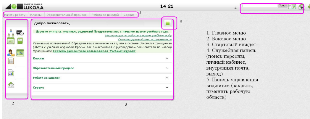
Рис. 3. Интерфейс пользователя.
