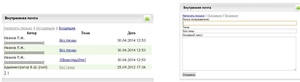
Рис. 11. Внутренняя почта.
