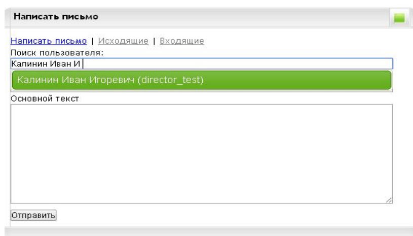
Рис. 12. Выбор адресата.
