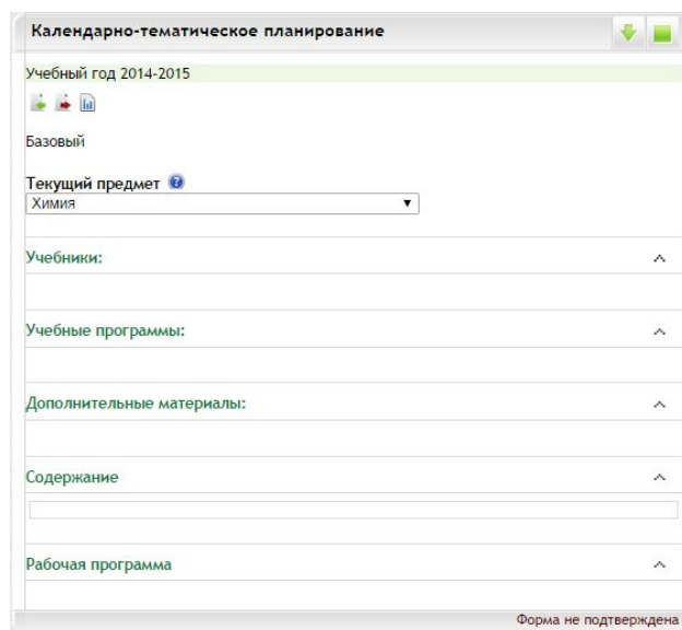
Рис. 6. Календарно-тематическое планирование
